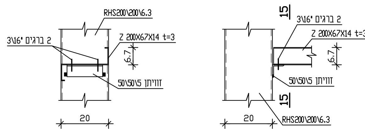
1:10 15-15 חתך 1:10 1 פגט
