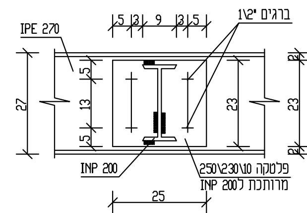
9A-9A חתך
