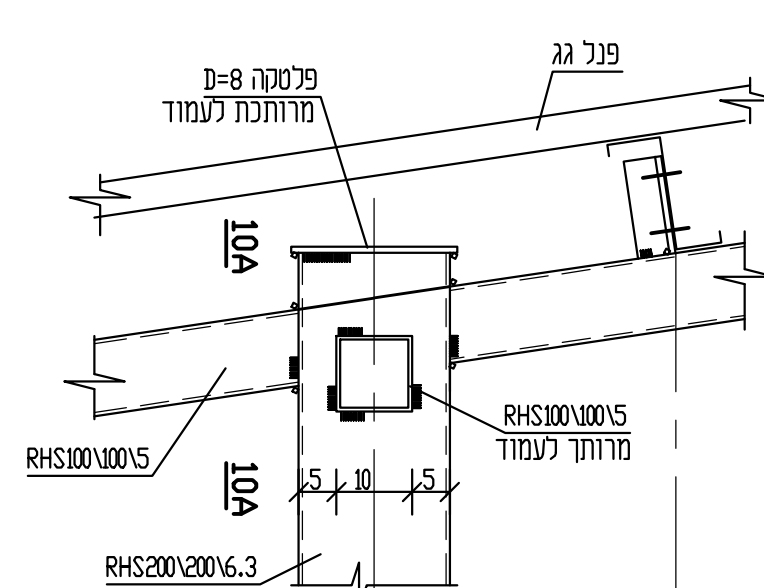
10-10 חתך
