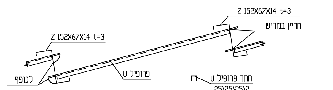
פרט חיבור בין מרישים
