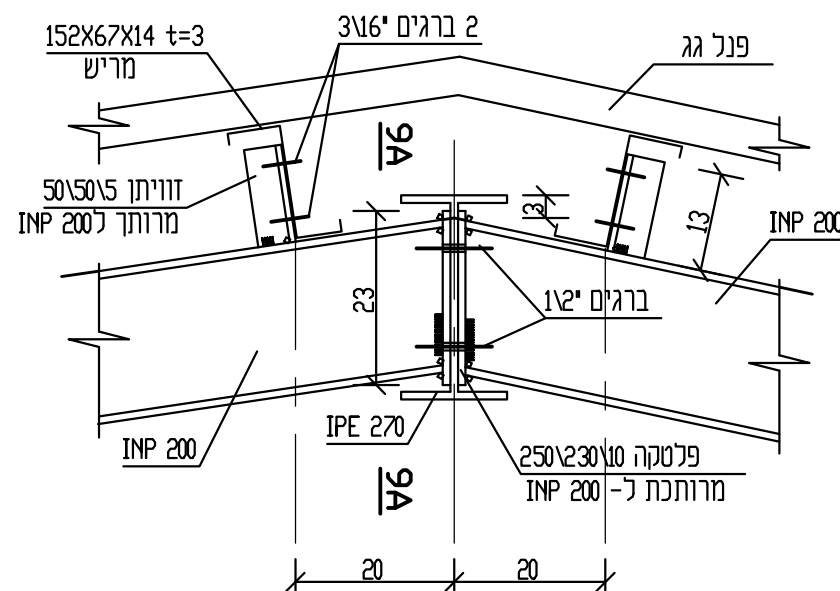
1:10 9-9 חתך
