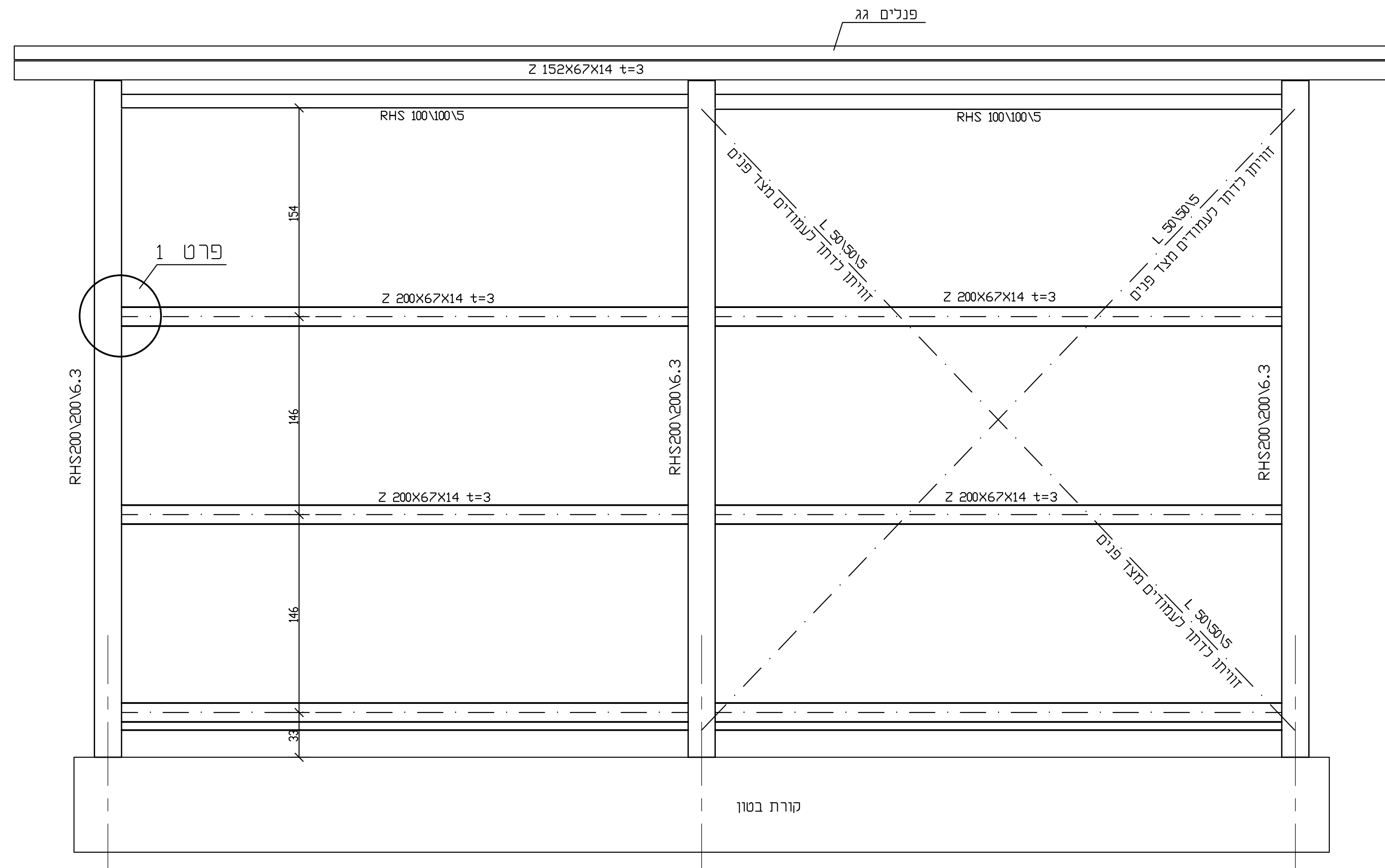
B-B חזית
