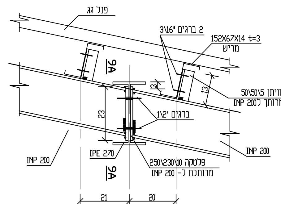
9*-9* חתך
