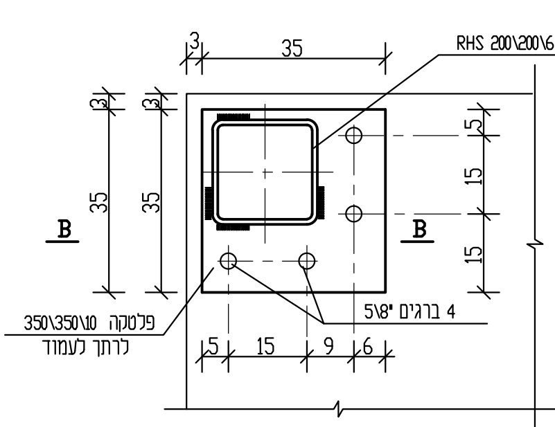
פרט חיבור עמוד פינתי עם רצפה
