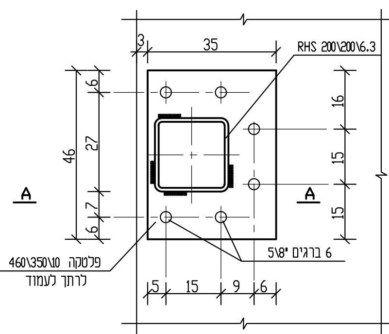
פרט חיבור עמוד עם רצפה
