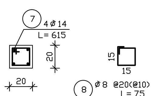
חתך טיפוסי של עמודים
