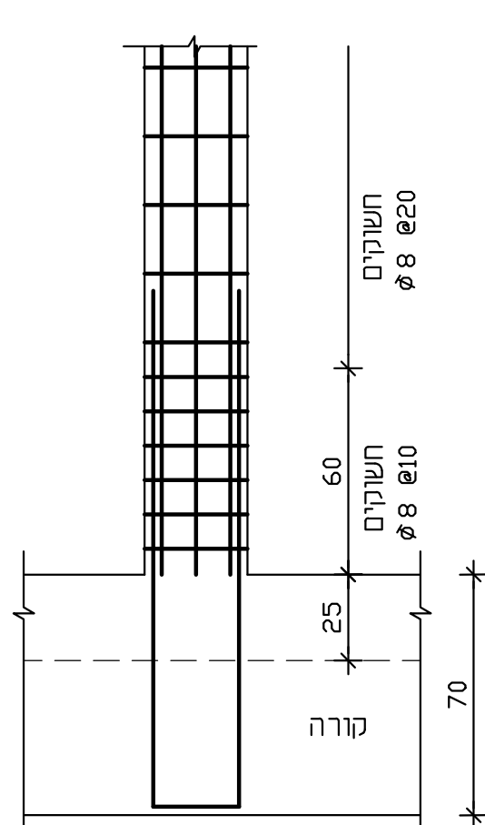
פרט חפיפה בין דיון העמוד
